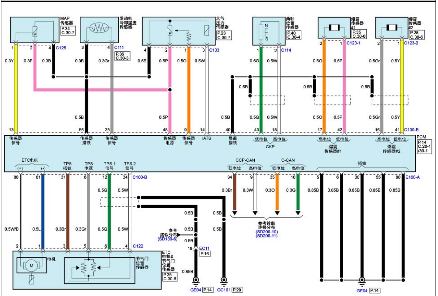
发动机控制系统(G6DH : LAMBDA II 3.3L GDI)(9)
